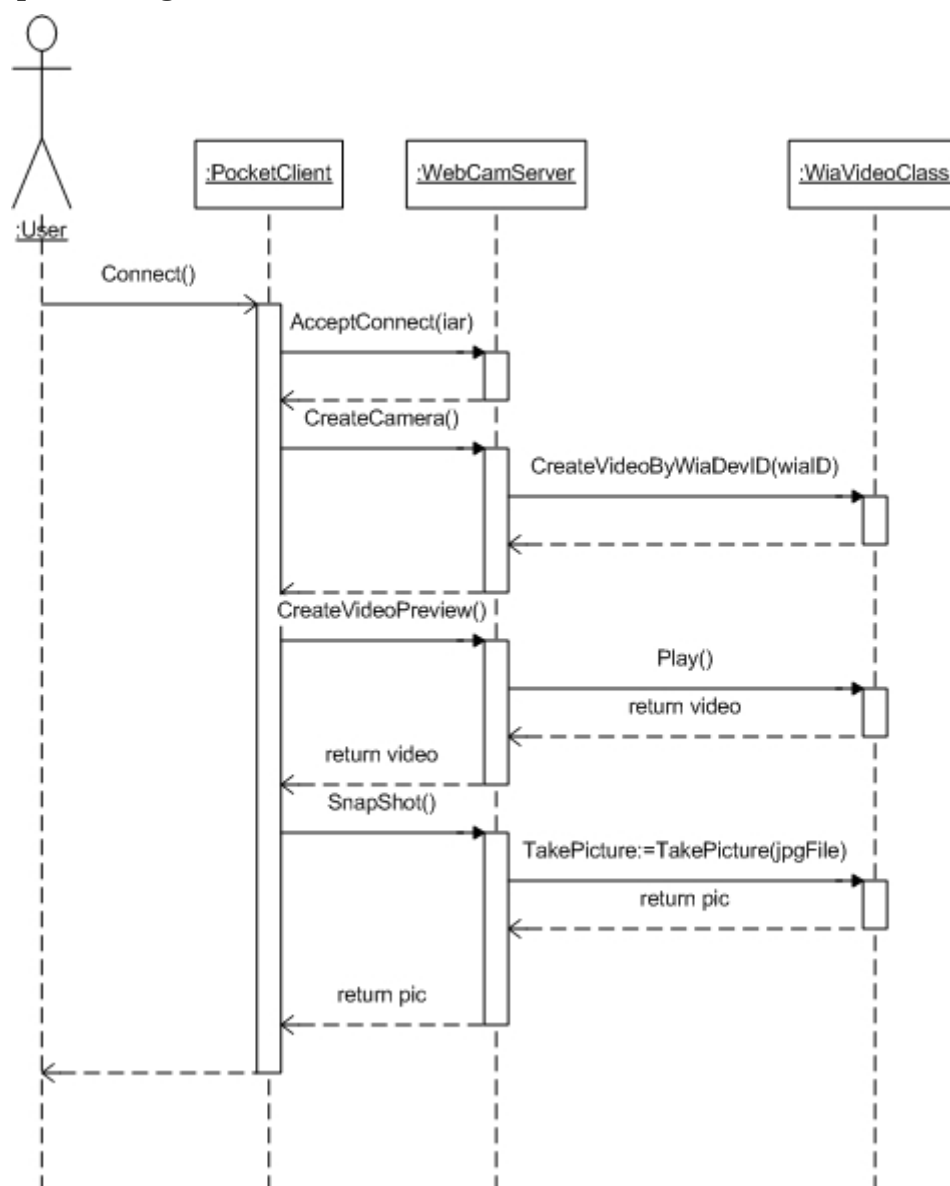
รูปที่ 8.4 Sequence Diagram แสดงการติดต่อระหว่าง Pocket PC กับเครื่องเซิร์ฟเวอร์ และแสดงผลภาพเคลื่อนไหวบน Pocket PC
